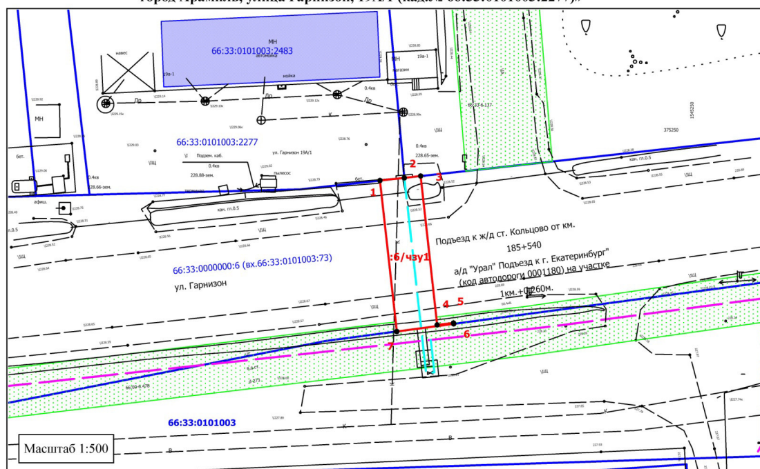
Схема расположения границ публичного сервитута в отношении части земельного участка с кадастровым номером 66:33:0000000:6 (вх. 66:33:0101003:73) для размещения «Газопровод высокого давления до границы земельного участка по адресу: Российская Федерация, Свердловская область, Арамильский городской округ, город Арамиль, улица Гарнизон, 19А/1 (кад.№ 66:33:0101003:2277)»
